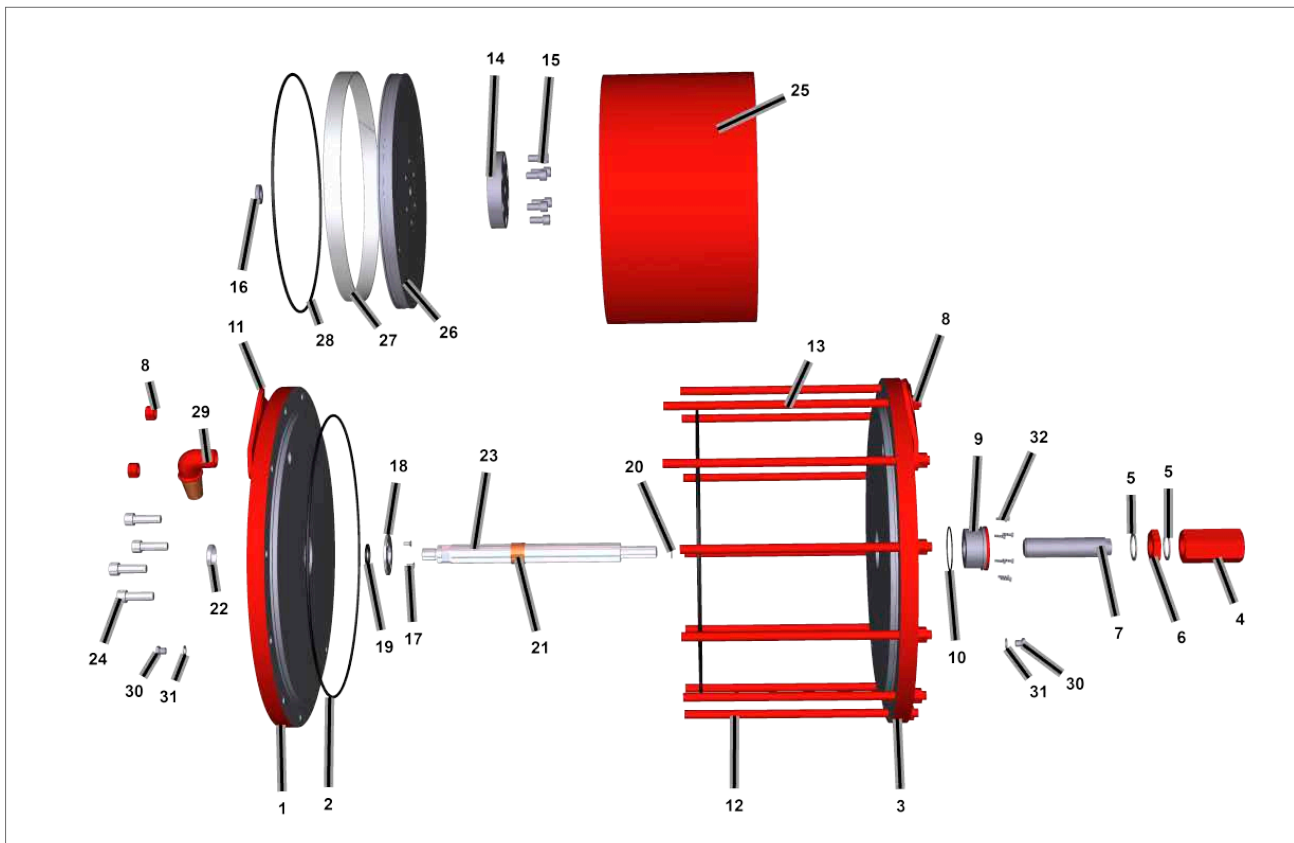
Fig 17.7 Vérin pneumatique
