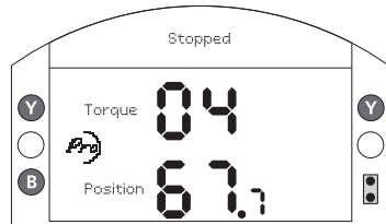
图 4.4.4 Torque (D) + Position 阀位 + 力矩数字显示
