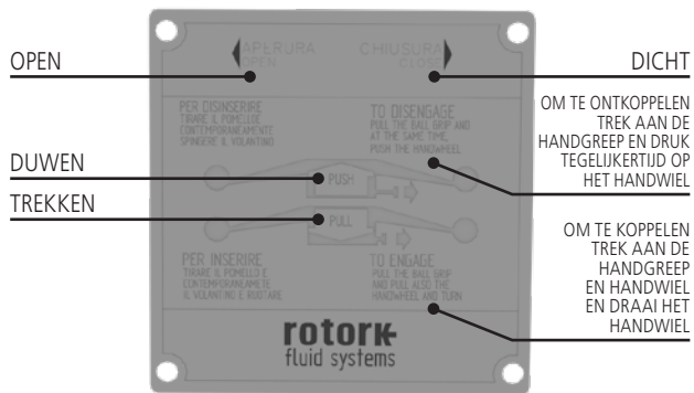
Afb 12.9 Plaatje met instructies voor handmatige controleovername MHD
