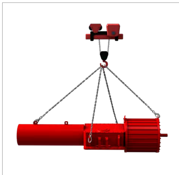
Afb 7.3 Optillen (enkelwerkende aandrijving maat 200 - 350)
