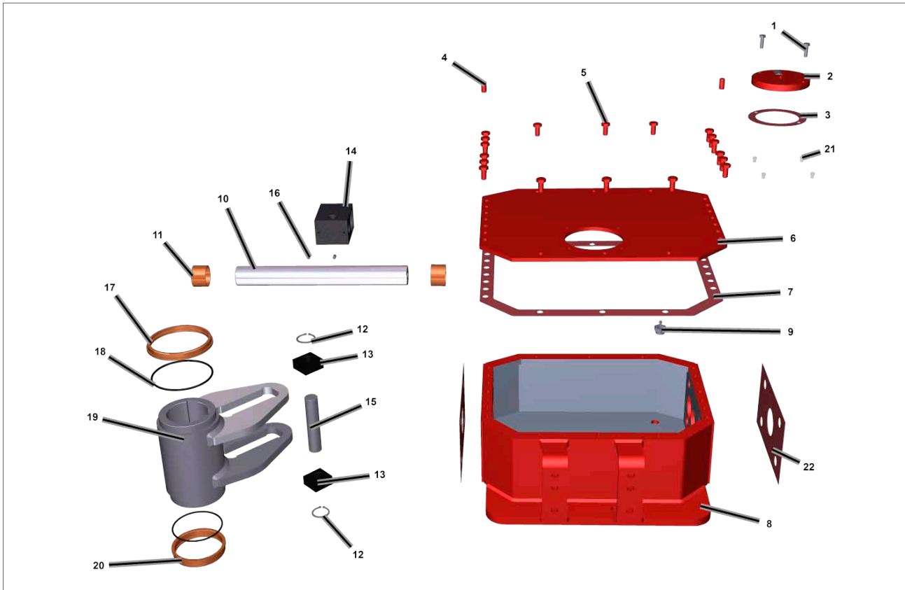
Afb 17.3 Centrale romp (gelast) (Aandrijving maat 065, 85, 100, 130, 161, 350)
