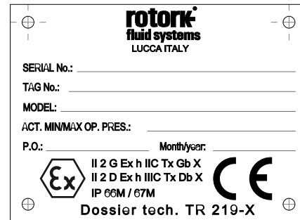
Afb 5.1 Label aandrijving
