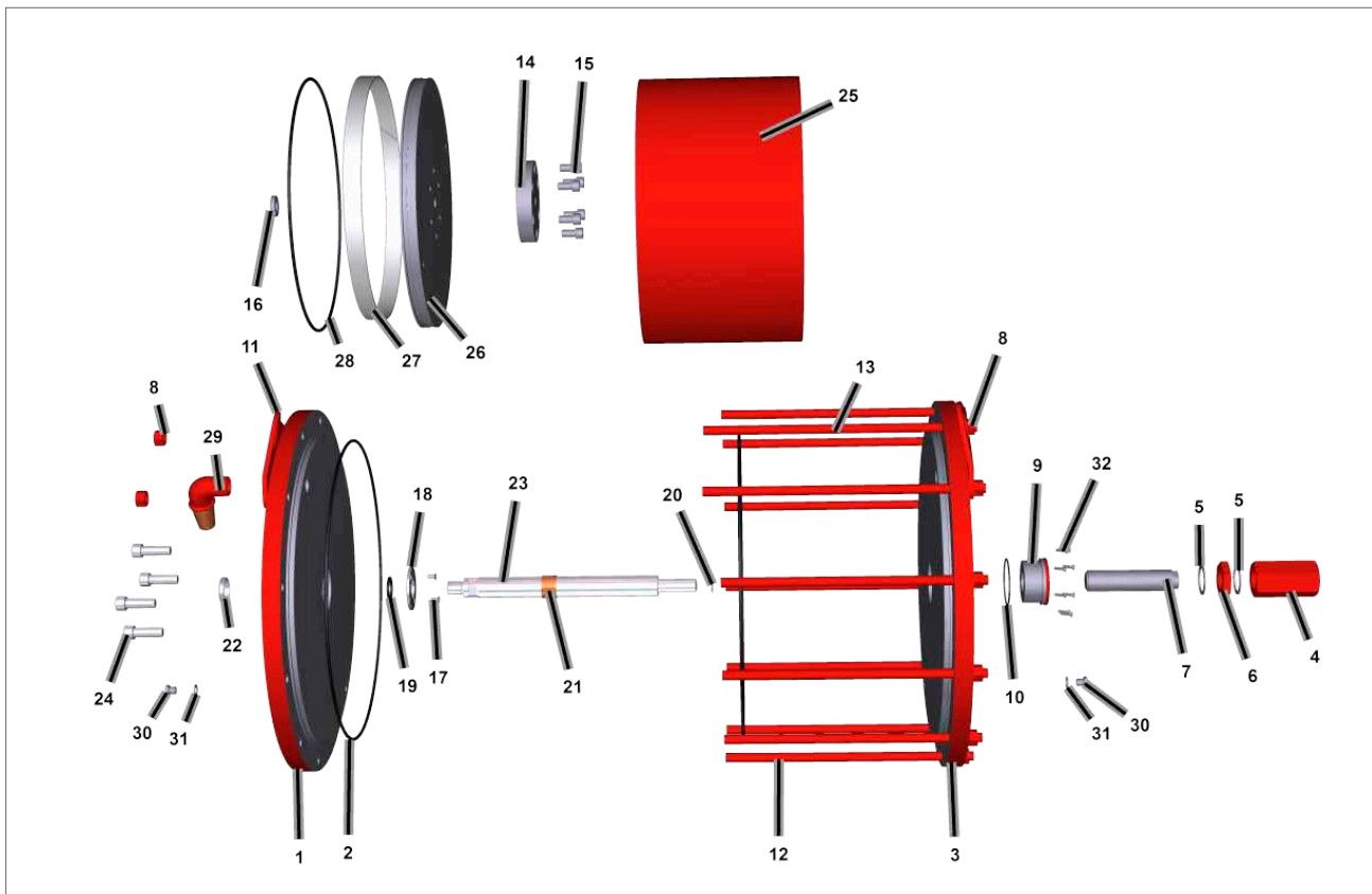
Afb 17.7 Pneumatische cilinder
