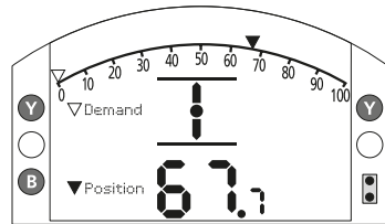
Fig. 4.4.5 Positioner (定位)
