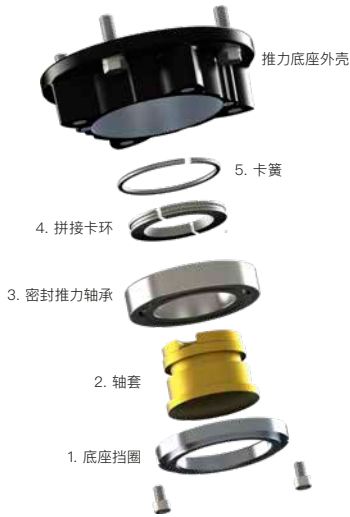
Fig. 5.1.2 底座拆解图
