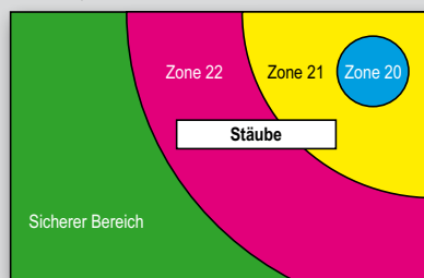
Beispiel eines typischen Zonenverlaufs, entstehend durch ein Getreidesilo mit Abfüllung in einem geschlossenen Raum.
