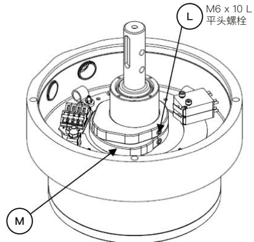
图7 - SPI调试: Ex e d变型和非危险区域用变型的可调零件
