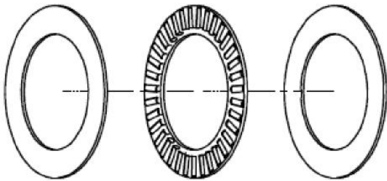
图2 - SPI 推力轴承的结构
