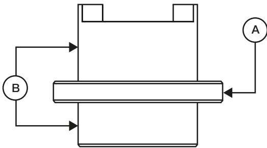
3 - SPI 输出轴套加工面/密封面
