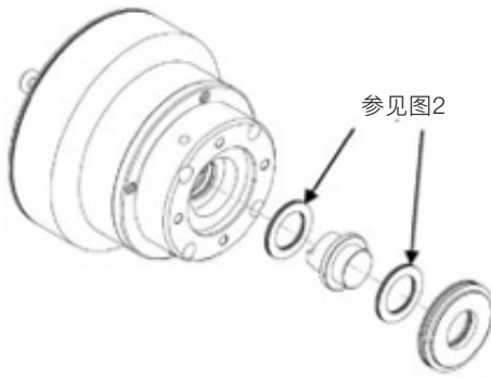
图1 - SPI 推力输出轴套组件
