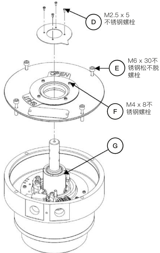
图5 - SPI调试：拆解
