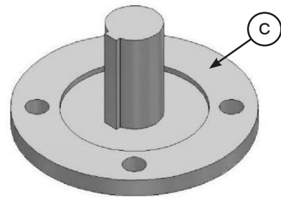
图4 - 密封胶定位面
