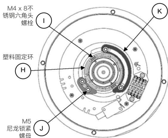
图6 - SPI调试: Ex i变型的可调零件
