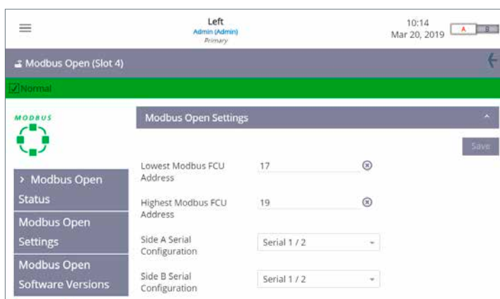
Fig. 6.24 Paramètres Modbus
