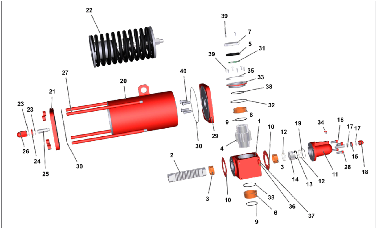
图 17.15 RH系列单作用执行机构
