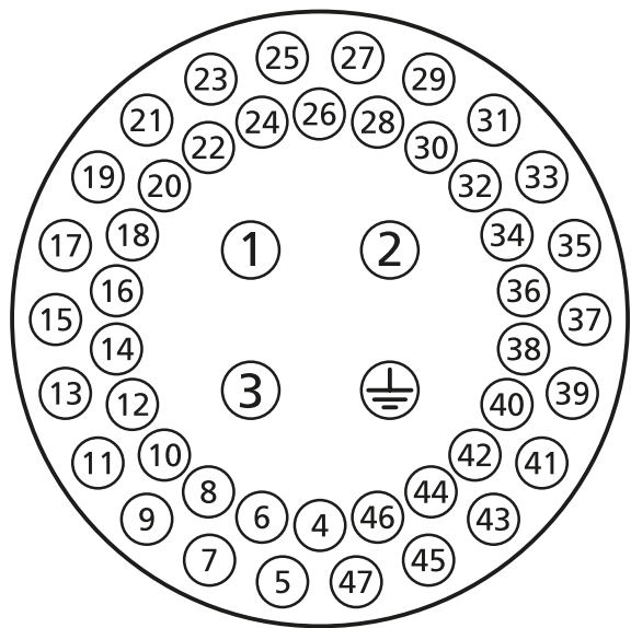
Fig. 7.1.1 Les numéros de bornes correspondent à ceux mentionnées sur le schéma de câblage
